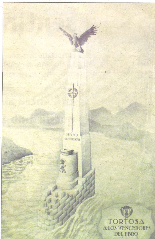
L'obelisc projectat per Barlett Zaldívar era de 26,5 metres d'alçada sobre un basament de 6,6x3,8 metres en planta, construït amb un nucli de formigó armat, paret de fàbrica de maó i revestiment exterior de pedra artificial. L'aliga que l'havia de coronar hagués tingut una alçada de 2,6 metres i hagués anat, amb bronze, amb les ales atirantades i ancorada, verticalment, al seu pedestal. / FOTO DE LÓPEZ DAUÍ DEL DIBUIX DEL MONUMENT DE BARLETT ZALDÍVAR
