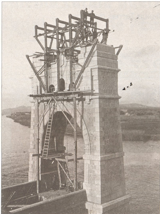
Imatge de la construcció d'una de les pilastres. / MUSEU TERRES DE L'EBRE
