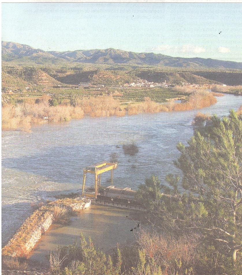
El azud de Xerta, donde parte del agua del Ebre va a los canales de la derecha y la izquierda. FOTO: JOAN REVILLAS
