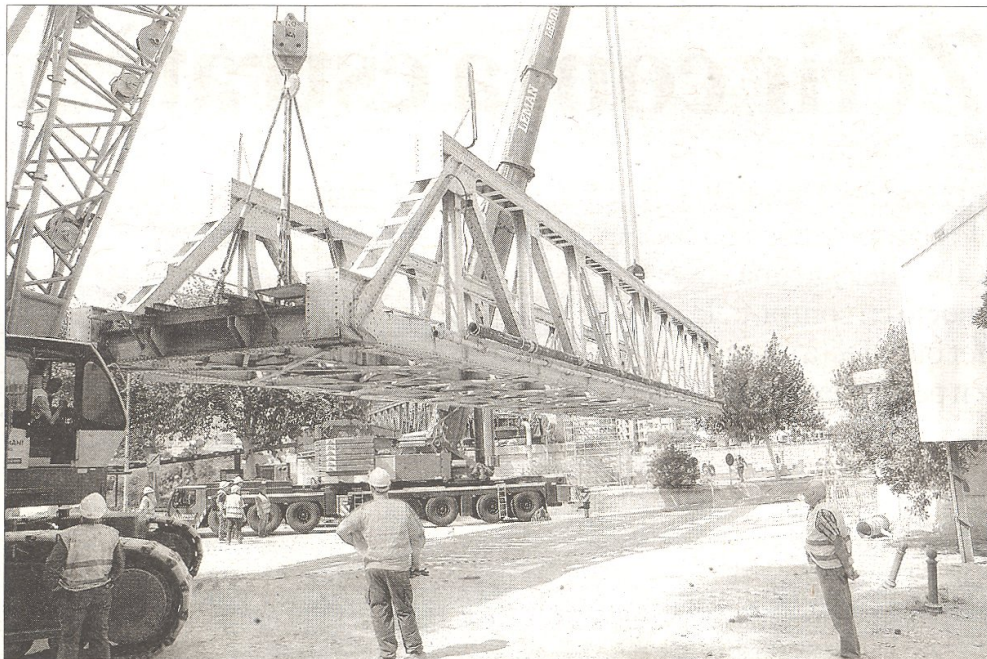
Les grues dipositen l'estructura metàl·lica del pont a l'aparcament del parc. FOTO: DT
