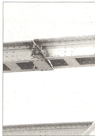
L'estructura es va haver de tallar per retirar-la. FOTO: DT
