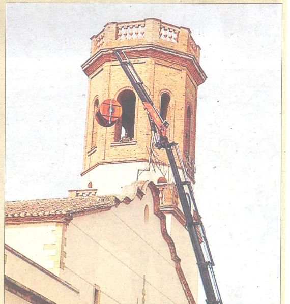
Maqueta de la matraca que més tard va ser construïda en mides molt superiors. A la dreta, la matraca, en el moment de ser pujada per una grua al campanar. Cal ressaltar que l'aparell fa un metre d'ample i l'ull del campanar per on va entrar medeix 1,10 metres. / V.C. / CEDIDA
