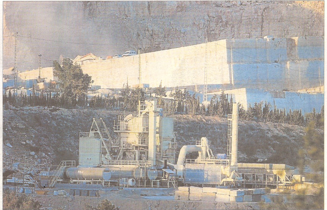
La planta d'aglomerat asfàltic, a Ulldecona. FOTO: JOAN REVILLAS
