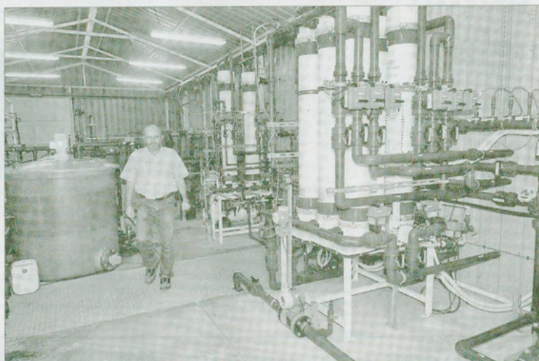
Planta pilot ELSA per assajar la millor tecnologia. El consorci va obrir ahir les portes de la planta pilot posada en servei l'any 2010 a l'Ampolla, per experimentar la millor tecnologia a fi d'eliminar les sals i sulfats de l'aigua de l'Ebre. La planta mantindrà la seva activitat fins a l'any vinent. FOTO: JOAN REVILLAS
